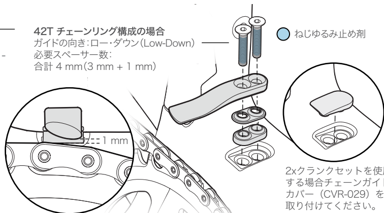
Low-Down ガイド取付方向
